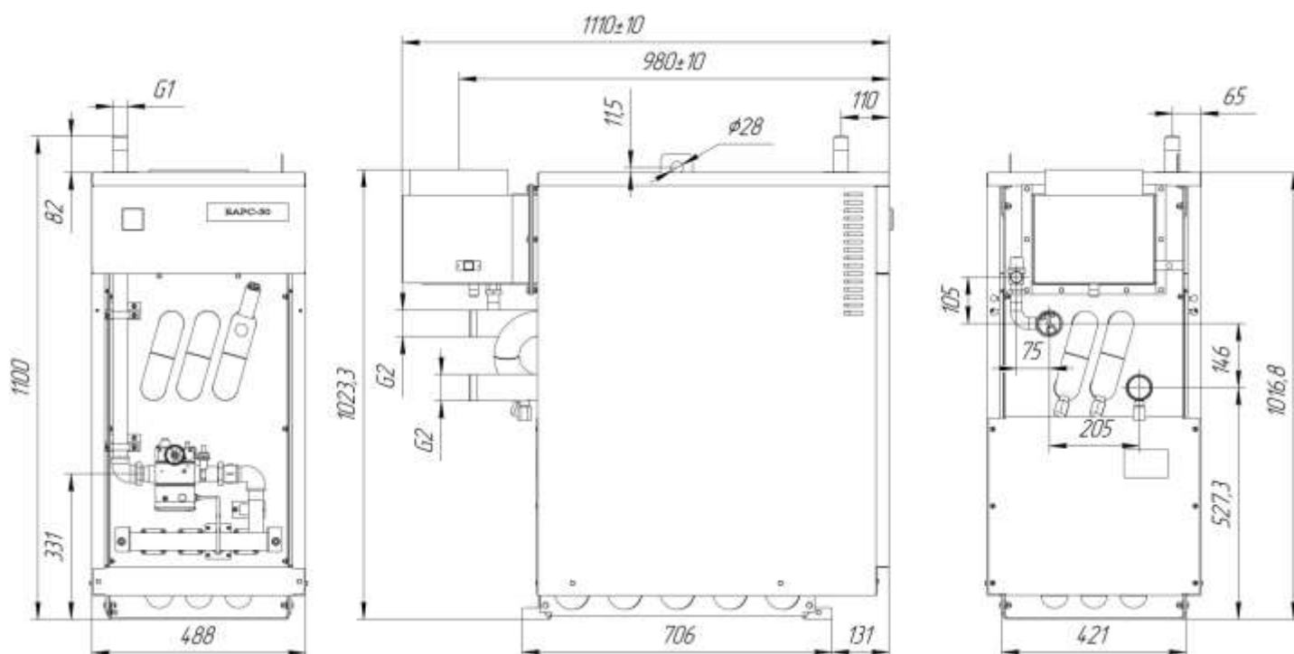
Рис. 1 Габаритные и присоединительные размеры
